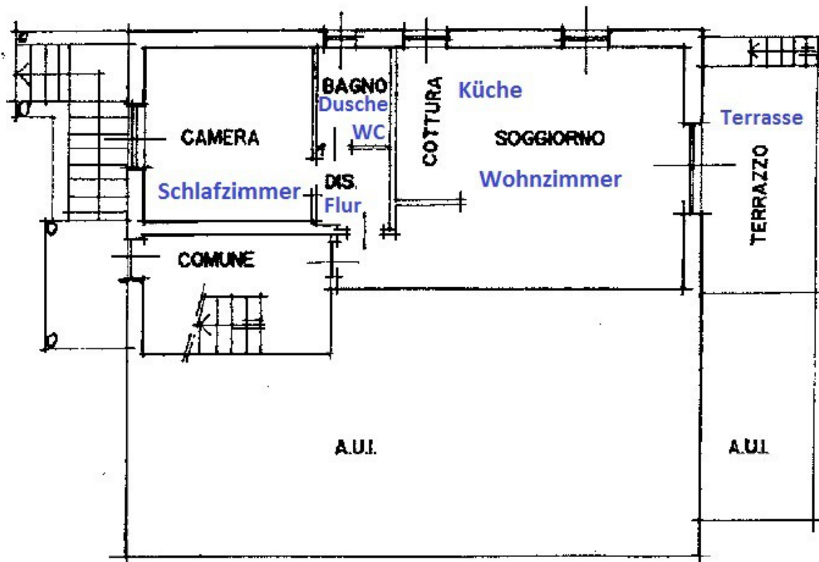
PIANO RIALZATO - H : 2.70
